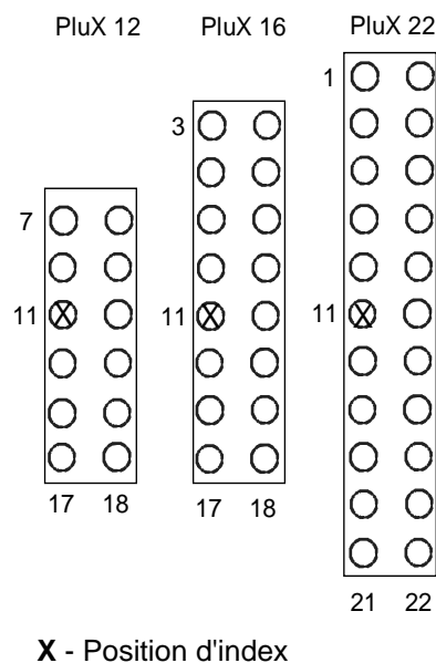
Fig. 2 : Aménagement des variantes des connecteurs PluX et définition de l'index, vue de dessus du support femelle)
