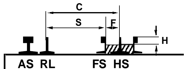
Weiche - Herzstückbereich
